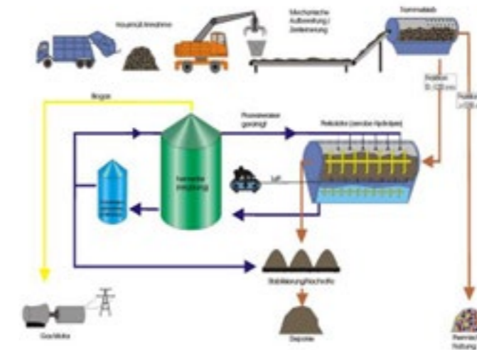
Anlagenschema MBA vereinfacht
